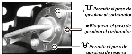
Imagen 10. Válvula de combustible.
