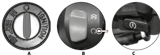
Imagen 29. Encendido de motor.
