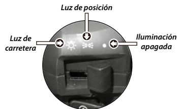
Imagen 3. Interruptor de luz delantera.
