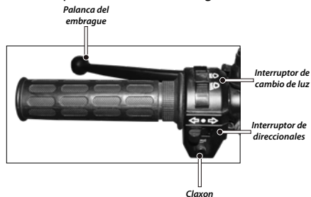
Imagen 4. Mando izquierdo.
