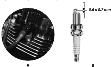
Imagen 17. Bujía.
