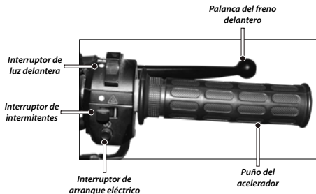
Imagen 1. Mando derecho.
