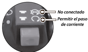
Imagen 4. Interruptor cortacorriente.
