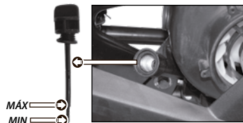
Imagen 13. Tapón-bayoneta del cárter.
