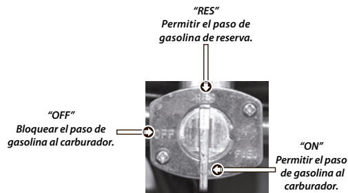
Imagen 9. Válvula de combustible.
