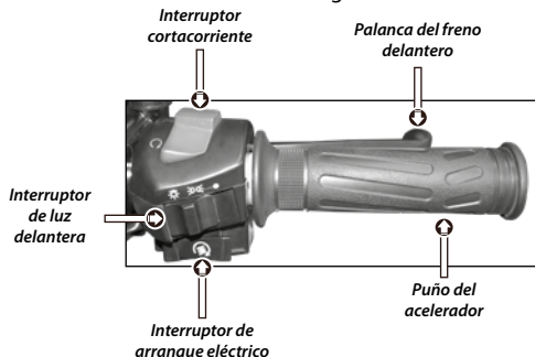
Imagen 1. Mando derecho.
