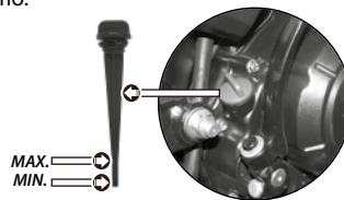
Imagen 15. Tapón-bayoneta del cárter.
