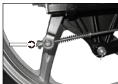
Imagen 24. Ajuste del pedal del freno trasero.
