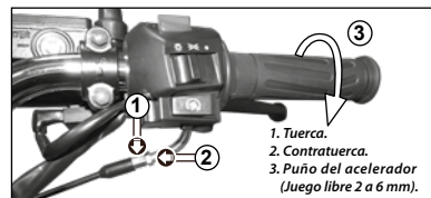
Imagen 19. Ajuste del puño del acelerador.
