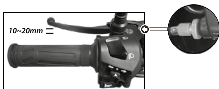
A B Imagen 20. Ajuste de la palanca del embrague.
