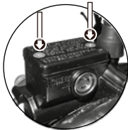
Imagen 26. Completar el nivel del líquido de freno.
